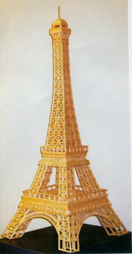
„Eiffelturm“, aus Samba-Leisten 5 x 5 mm. Größe: 40 cm x 40 cm x 102 cm. Inga-Louisa Laux, Gymnasium Marienschule, Krefeld, Kunsterzieher Werner Lichtenberg.
